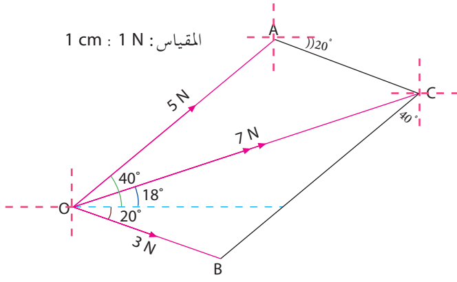
شكل 3 - 14 جمع المتجهات بقانون متوازي الأضلاع
