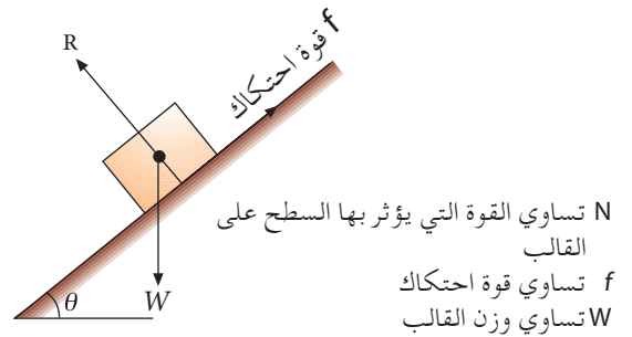
شكل 3-27 قالب موضوع على سطح مائل
