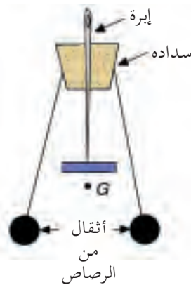
شكل 5 - 26 لعبة توازن : موازنة إبرة
