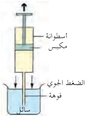
شكل 4 - 7 الحاقنة
