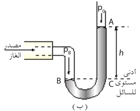
شكل 7-20 مانومتر لقياس ضغط مصدر الغاز
