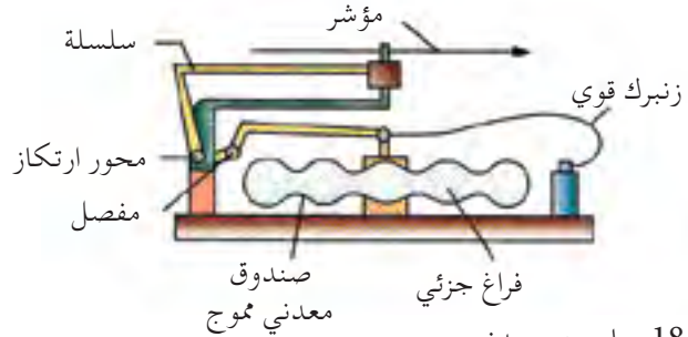
شكل 7 - 18 بارومتر معدني
